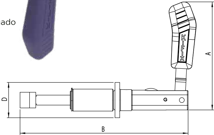
Grampo recuado
